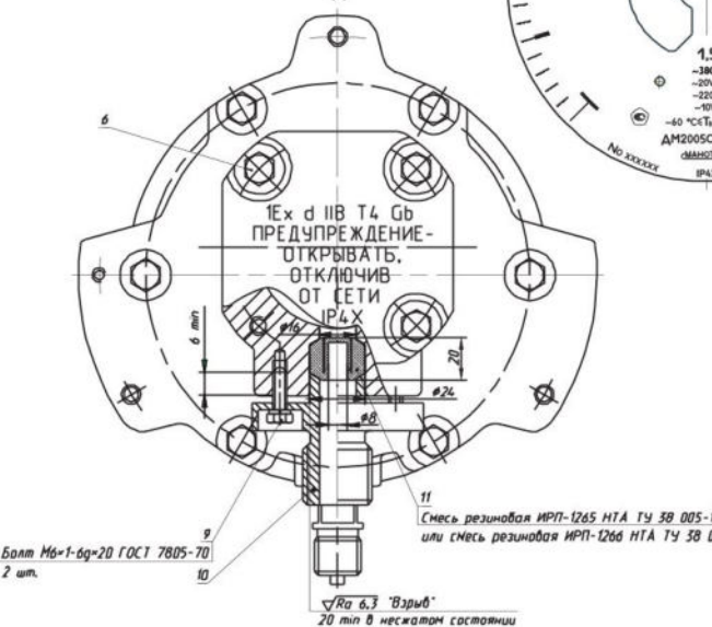
Рисунок В.1 - Чертеж средств взрывозащиты для ДМ2005СГ1Ех, ДВ2005СГ1Ех, ДА2005СГ1Ех (ИР4Х)
