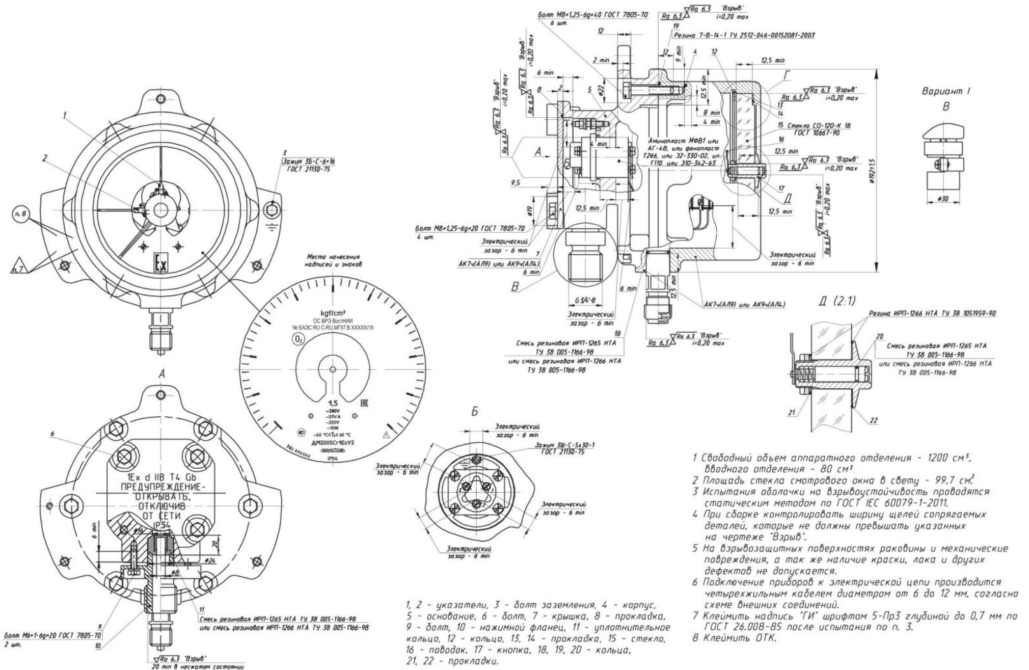
Рисунок В.2 - Чертеж средств взрывозащиты для ДМ2005Сг1Ех, ДВ2005Сг1Ех, ДА2005Сг1Ех (IP54)
